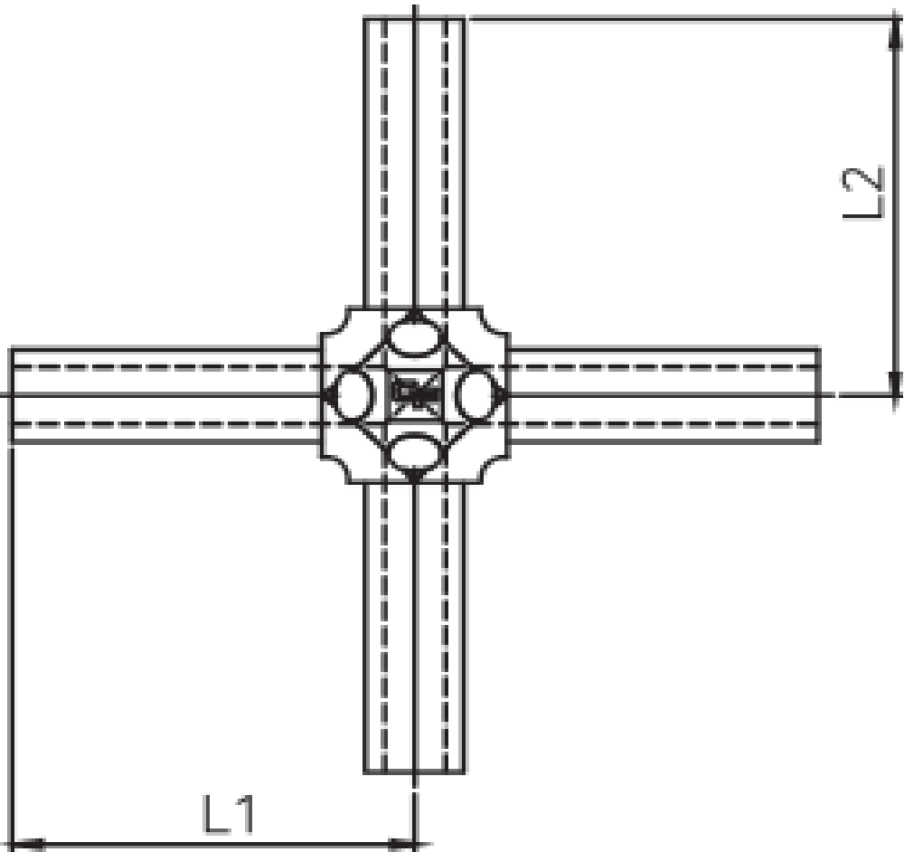
十字通（单位: mm）
